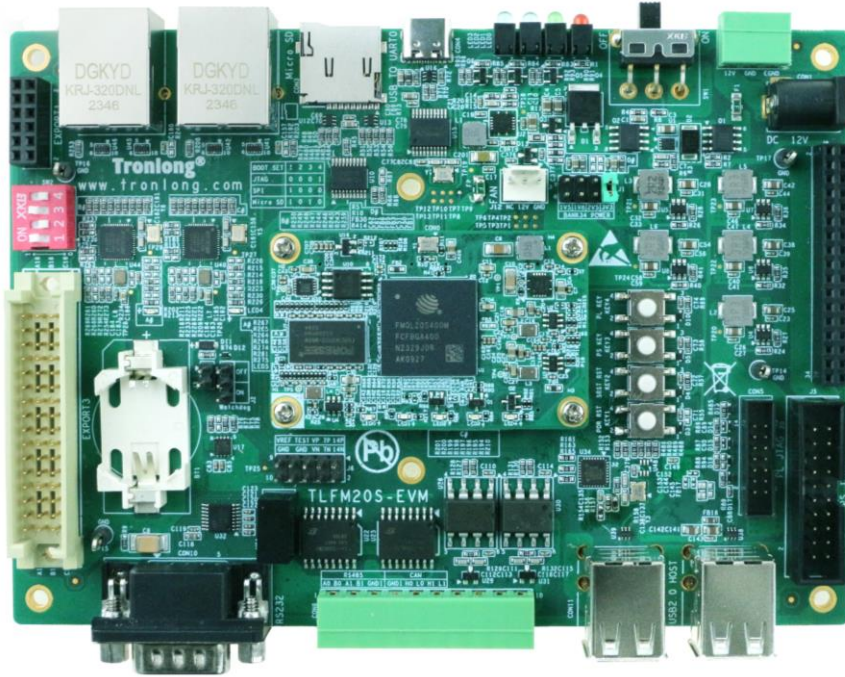
图 1 评估板正面图
