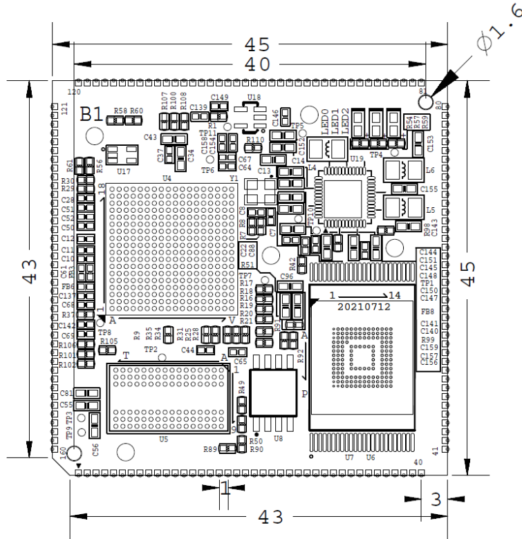
图 8 核心板机械尺寸图（顶层透视图）
